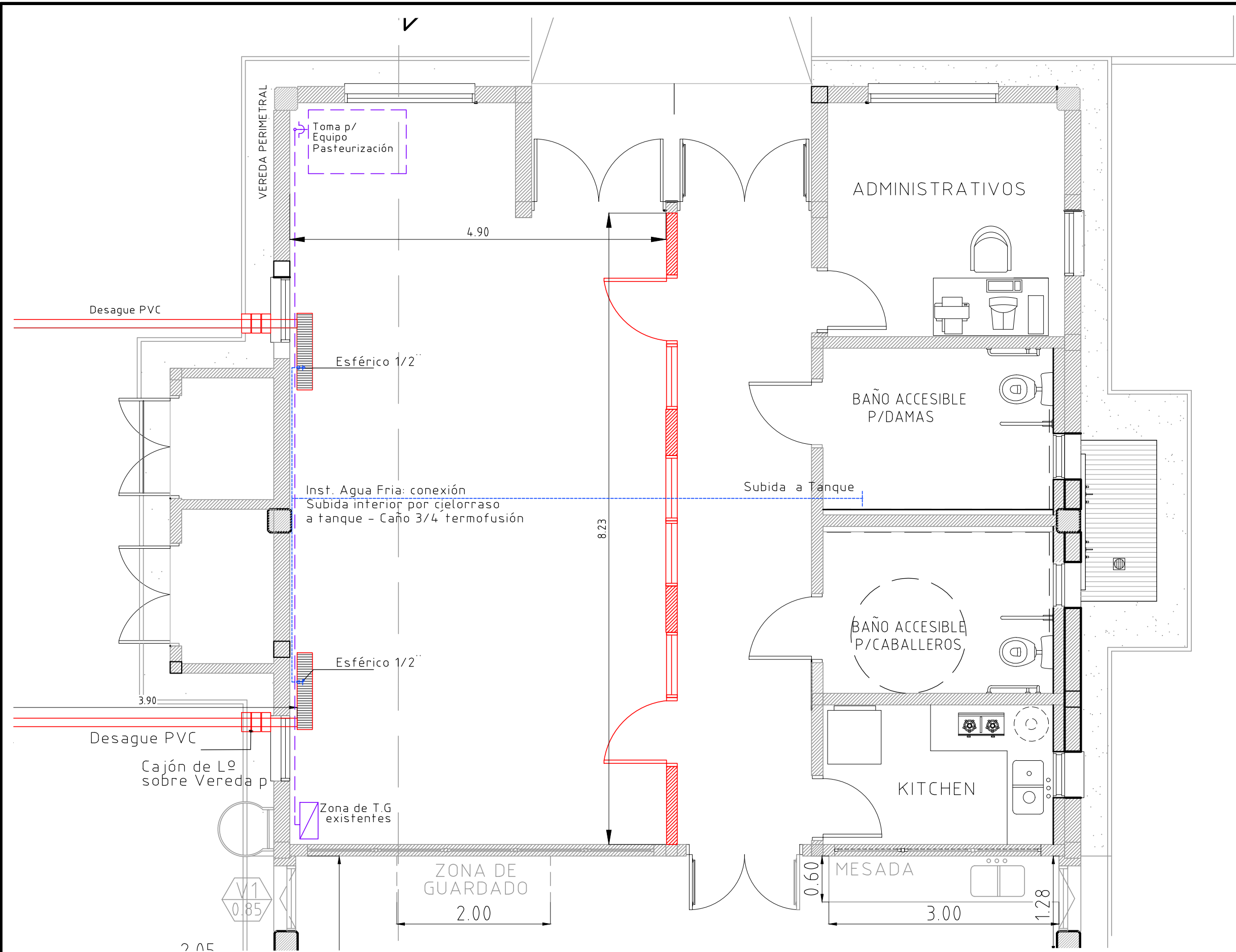
PLANTA GENERAL
