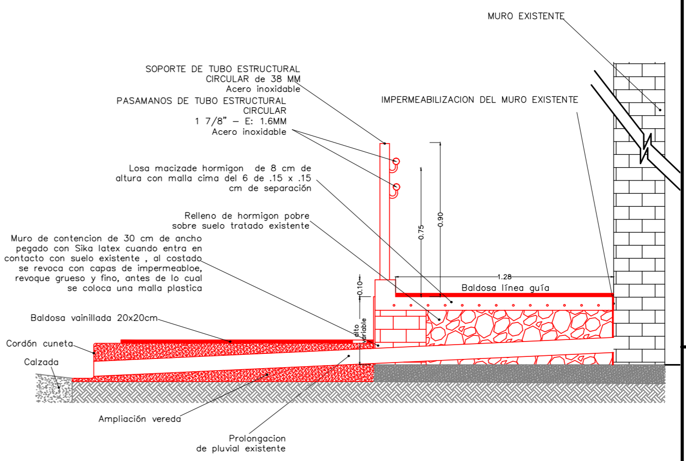
DETALLE CONSTRUCTIVO
